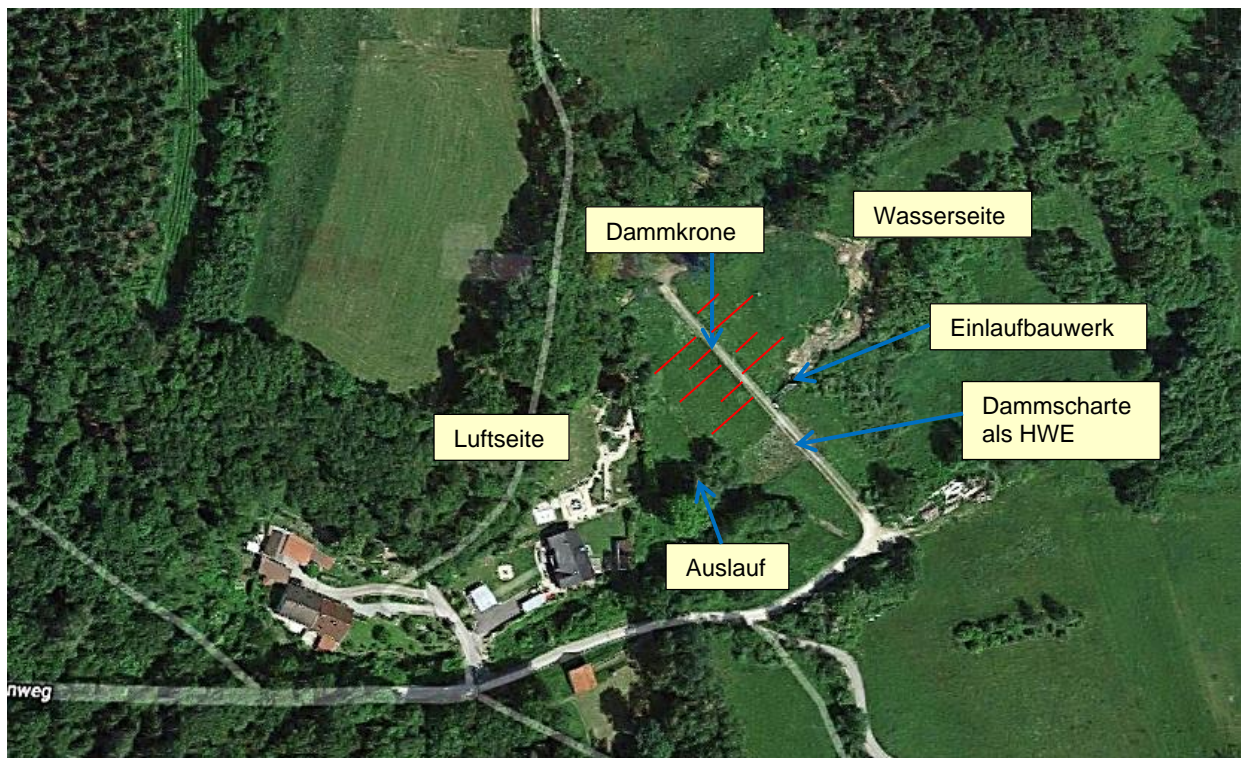
Abbildung 2: Luftbild HRB Aubach (Quelle: Google Maps)
